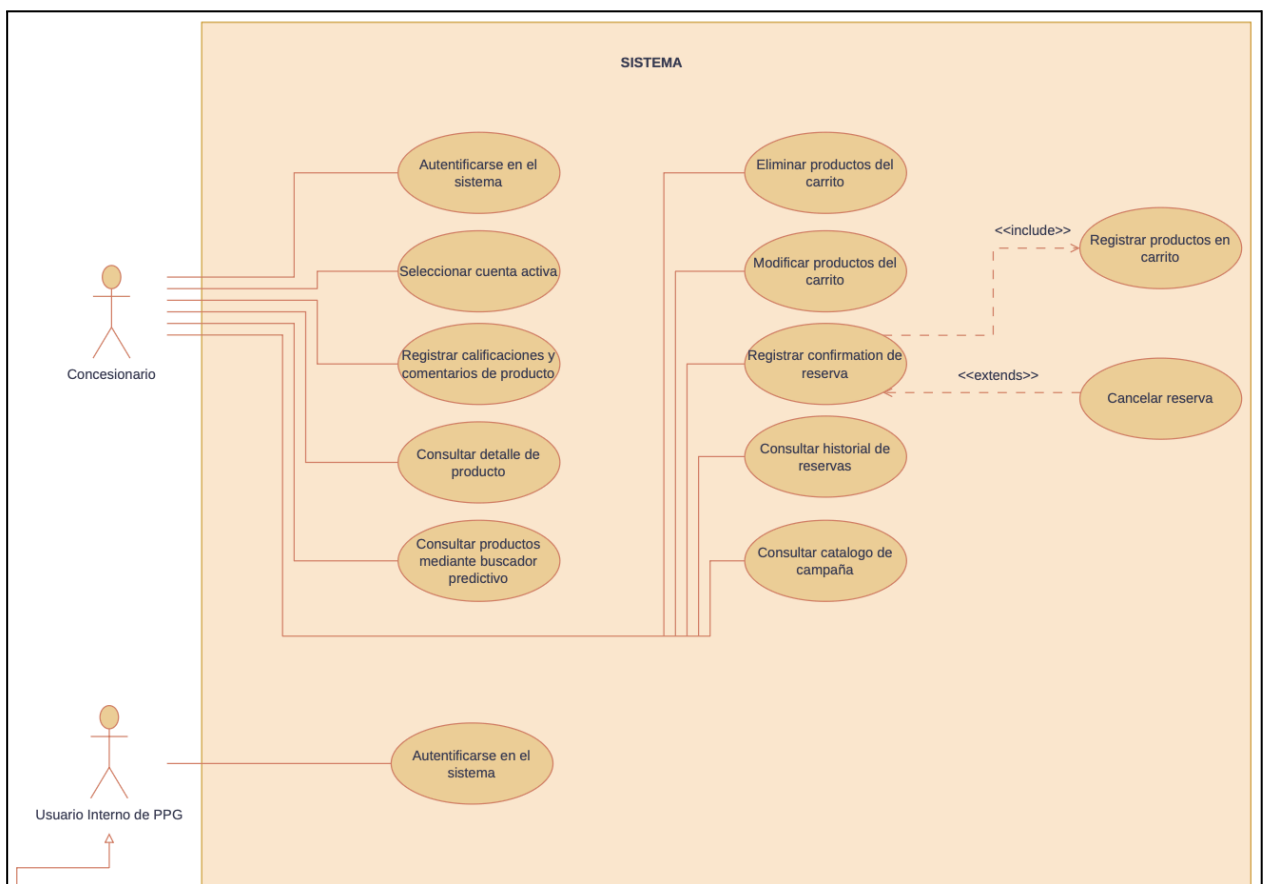
Fig. 3. Diagrama de casos de uso - Parte 1
