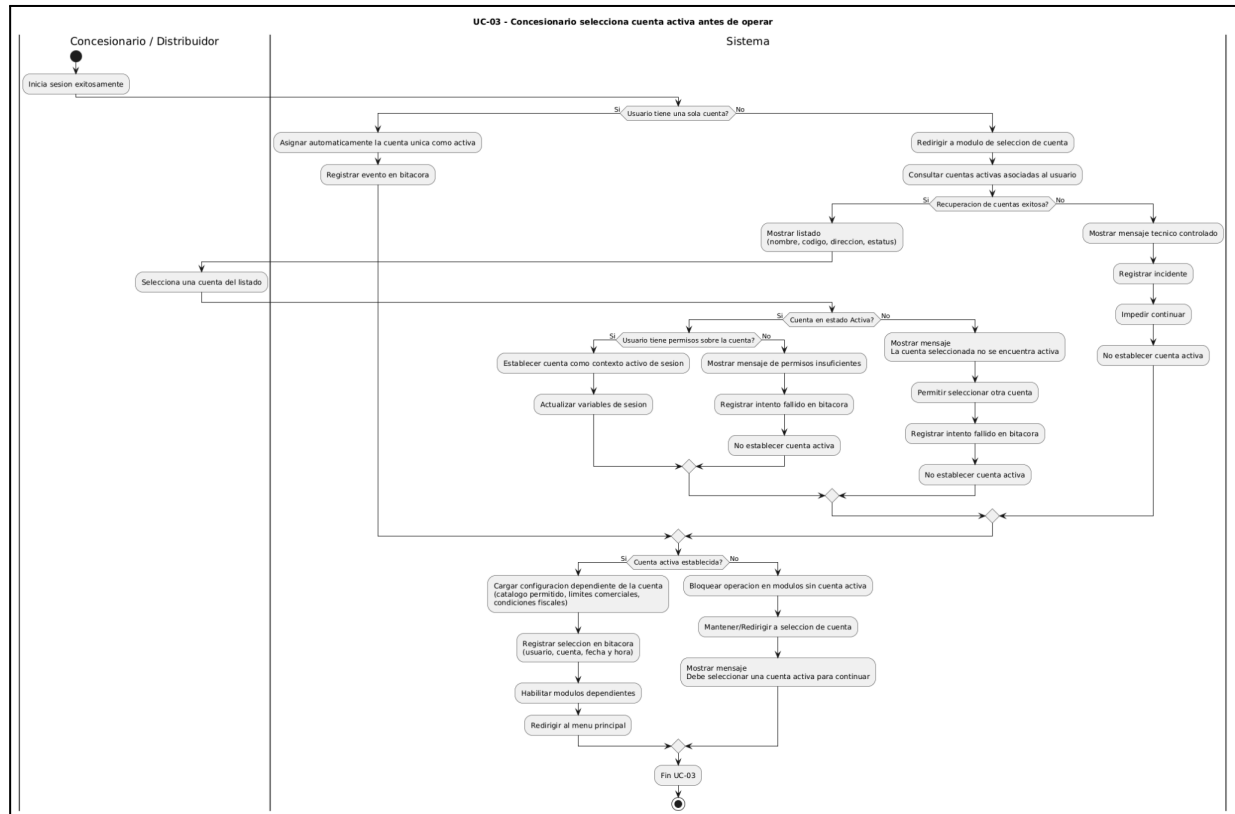
Fig. 7. Diagrama de actividad CU-03
