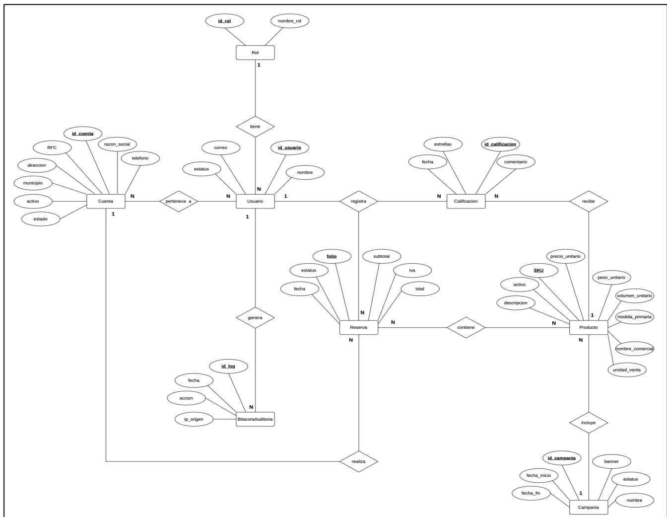
Fig. 11. Diagrama MER.
