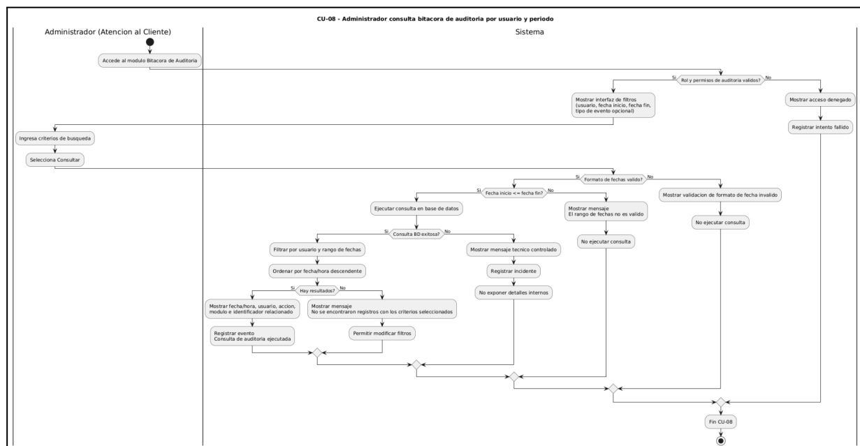
Fig. 10. Diagrama de actividad CU-08
