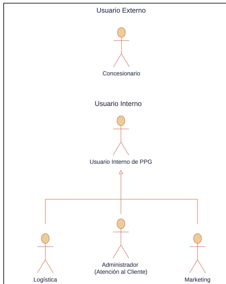
Fig. 2. Diagrama de casos de uso (jerarquía de actores)
