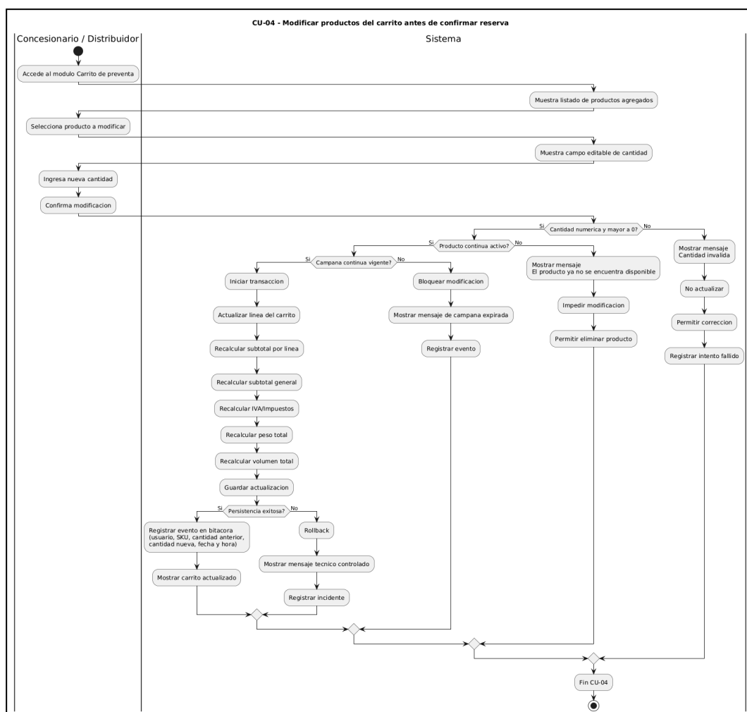
Fig. 8. Diagrama de actividad CU-04
