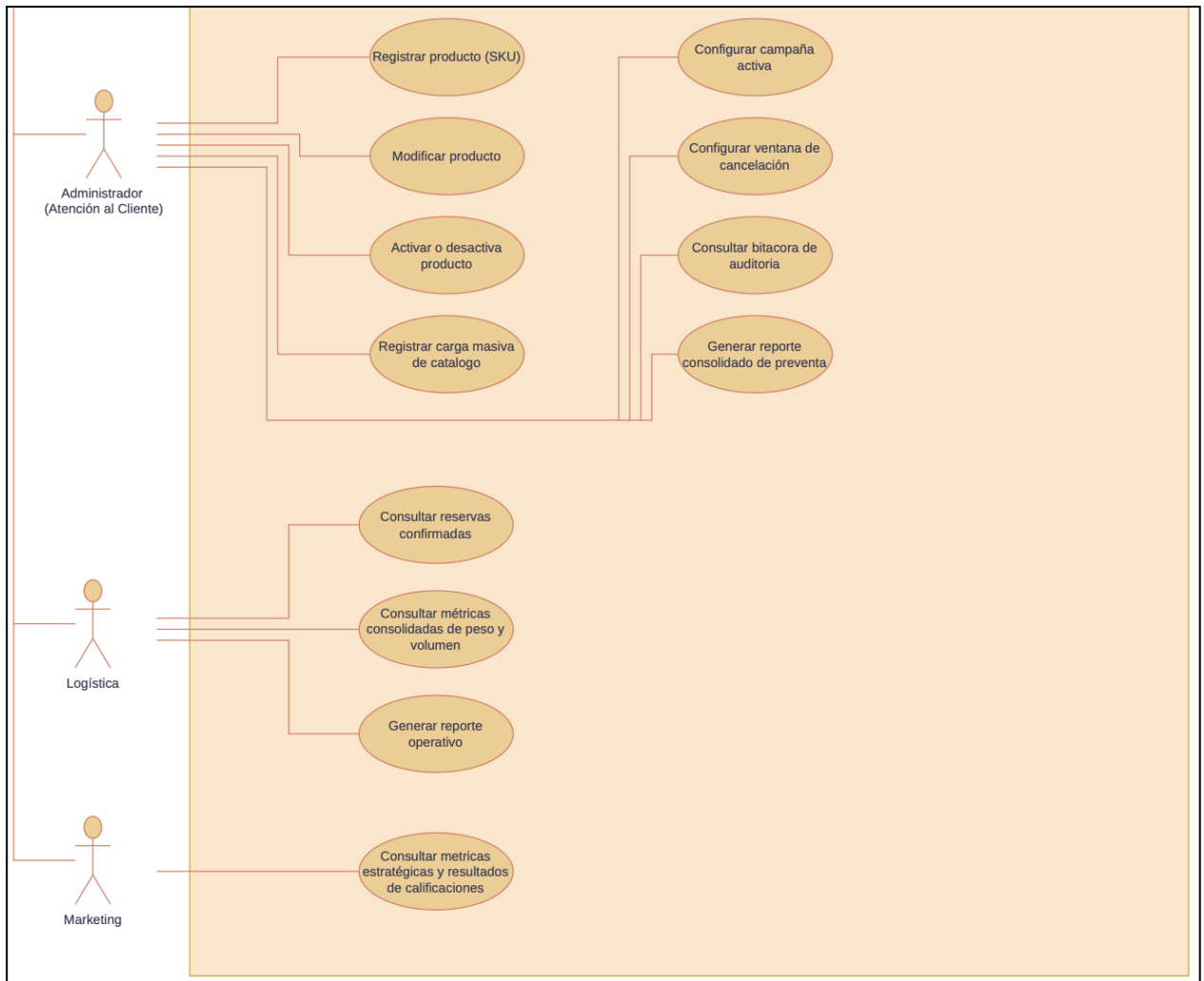
Fig. 4. Diagrama de Casos de Uso - Parte 2
